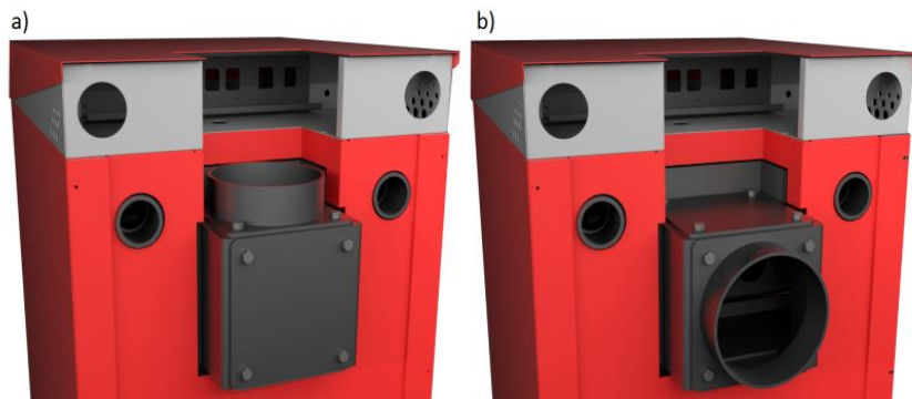
Rys. 17. Montaż króćca czopucha w kotłach KLIMOSZ DUO NG/EKO a) pozycja pionowa b) pozycja pozioma..
