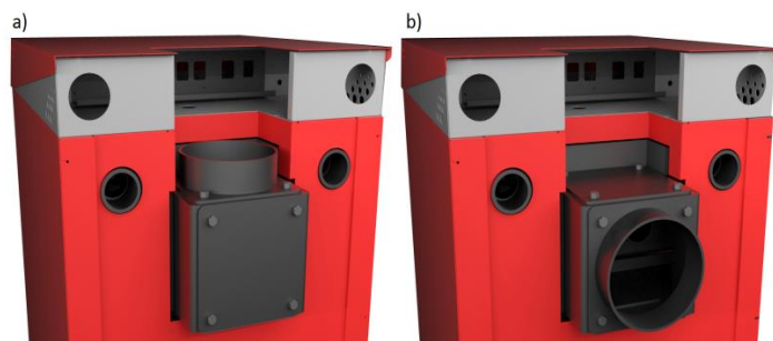
Rys.9. Montaż króćca czopucha w stalowych kotłach KLIMOSZ a) pozycja pionowa b) pozycja pozioma
