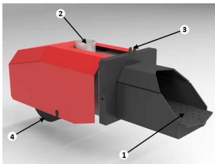
Rys.10 Palnik peletowy.
