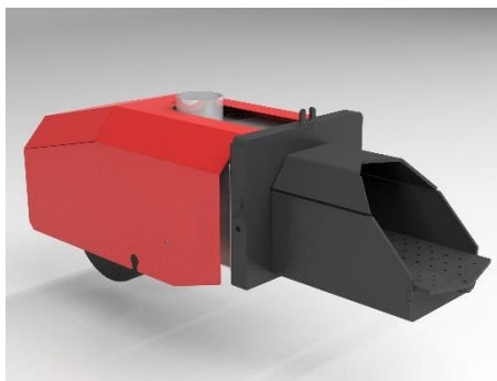
Rys 8. Wygląd palnika peletowego kotłów małej mocy.
