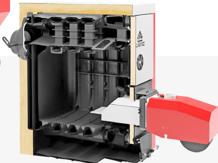
Rys. Przekrój kotła WALLY 22 po rozbudowie o zestaw ZPP.
