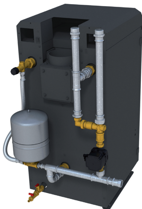
Przykład grupy bezpieczeństwa oraz grupy z zaworem termostatycznym dla kotła FRONTAL.
