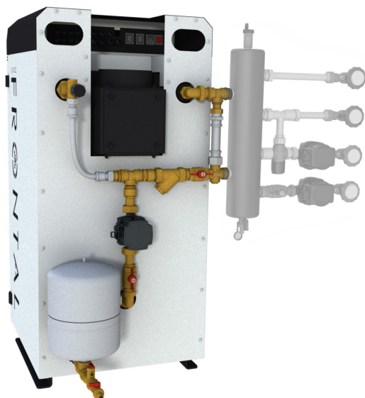
Przykład grupy bezpieczeństwa oraz aktywnej grupy ochrony powrotu dla kotła FRONTAL.
