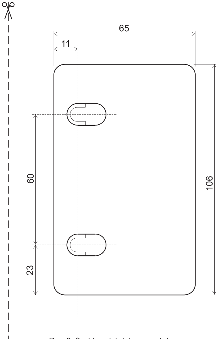
Rys. 2 Szablon ułatwiający montaż
