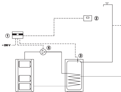
2. Podłączenie regulatora do instalacji z pompą ładującą podgrzewacz ciepłej wody użytkowej
