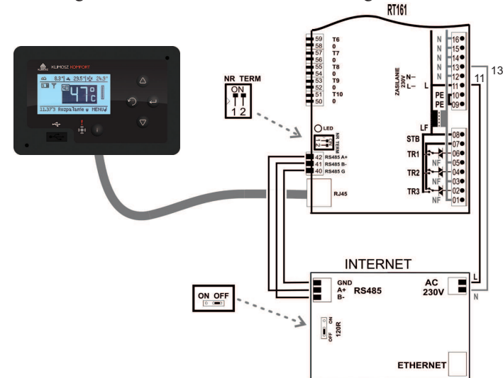
Rys.Int-2: Połączenie magistrali RS485 do modułu internetowego umieszczonego w pobliżu modułu wykonawczego RT161 (odległość do 50cm)
