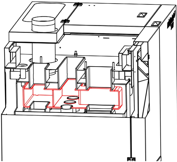
Krok 5 - Przez odsonięte kanały oczyścić komory rozprężne.
