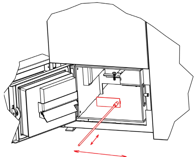
Krok 10 - Za pomocą czyszczaka oczyścić dno wymiennika.
