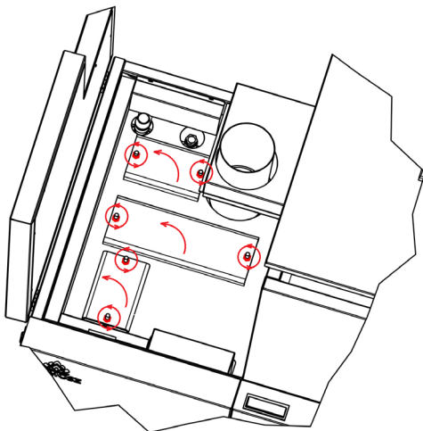
Krok 2 - Odkręcić nakrętki pokryw. Zdjąć pokrywy.
