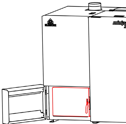
Krok 7 - Otworzyć dolne drzwi komory spalania.
