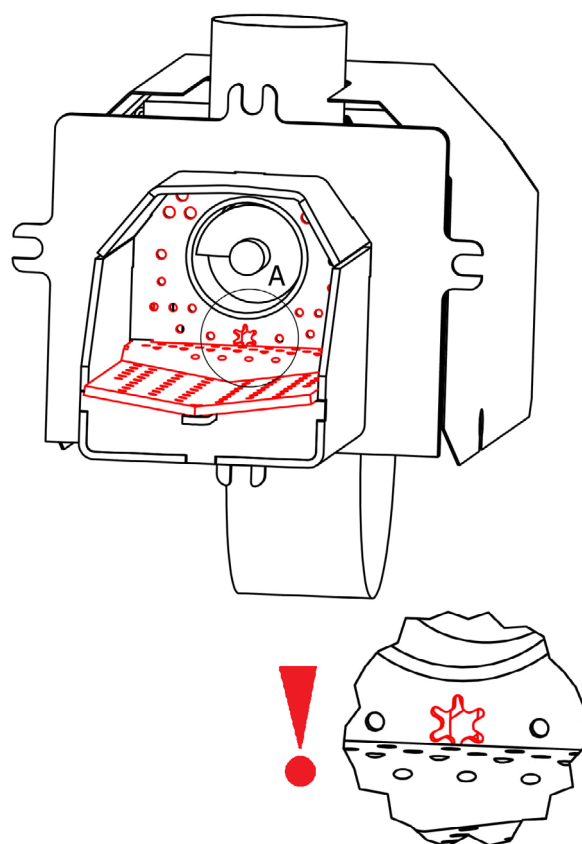
Krok 5 - Sprawdzić/oczyścić elementy palnika (otwory powinny być drożne). W szczególności sprawdzić miejsce działania zapalarki!
