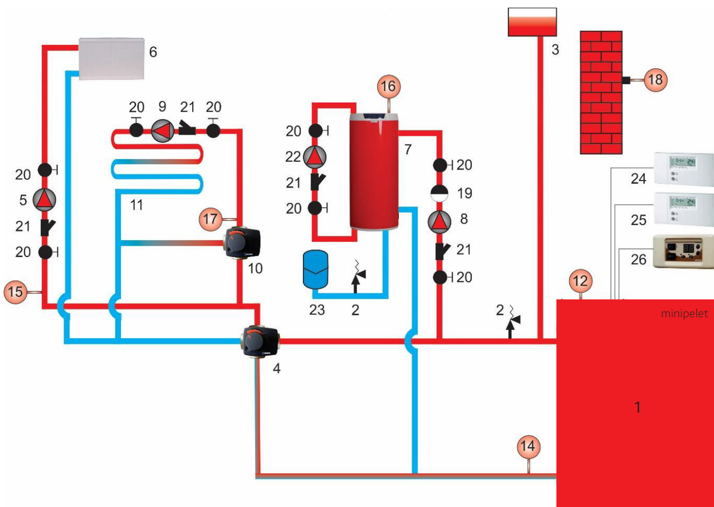
Rys. Schemat poglądowy montażu kotła w układzie otwartym z dwoma obiegami grzewczymi
