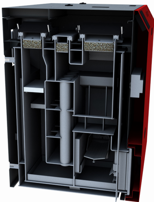
Rys. Przekrój kotła
