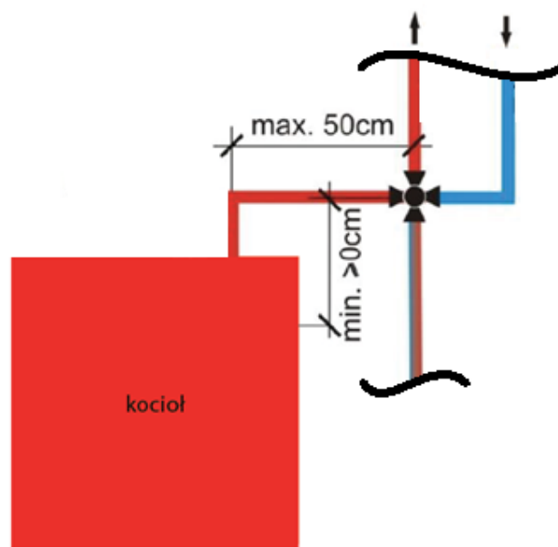
Rys. Schemat poglądowy umiejscowienia zaworu czterodrogowego.
