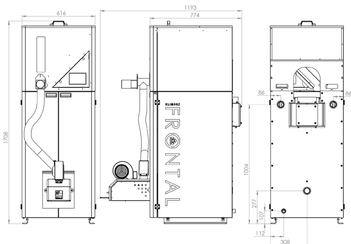
Frtional 10-18 kW, w wersji z zewnętrznym zasobnikiem
