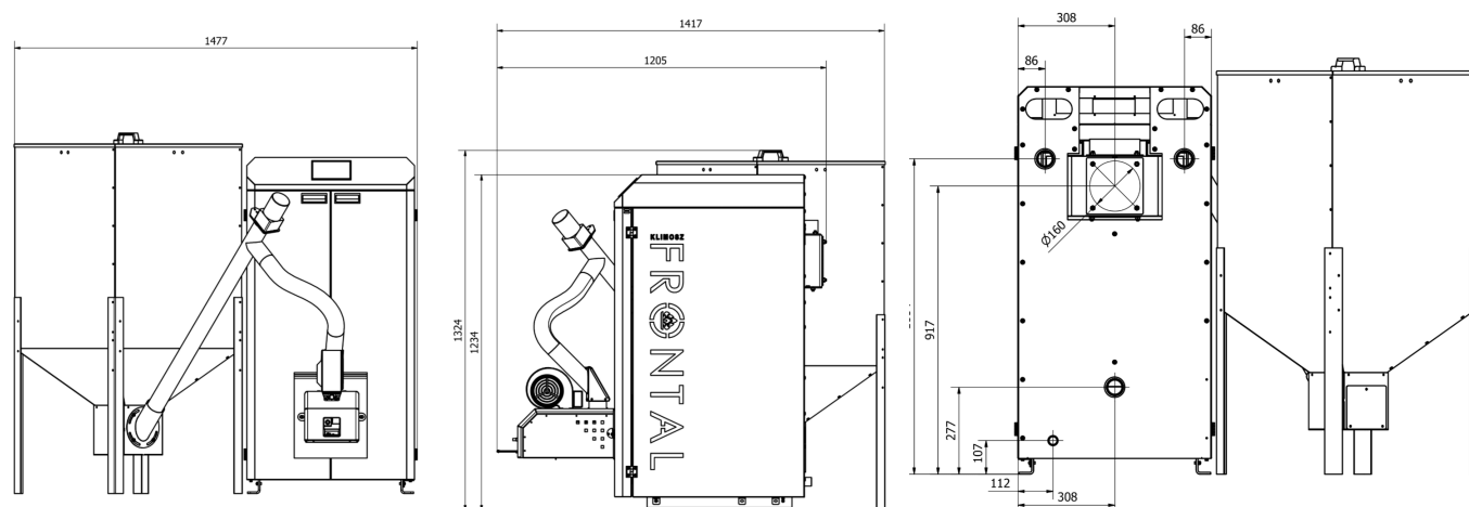
Frttonal 20-35 kW, w wersji z zewnętrznym zasobnikiem
