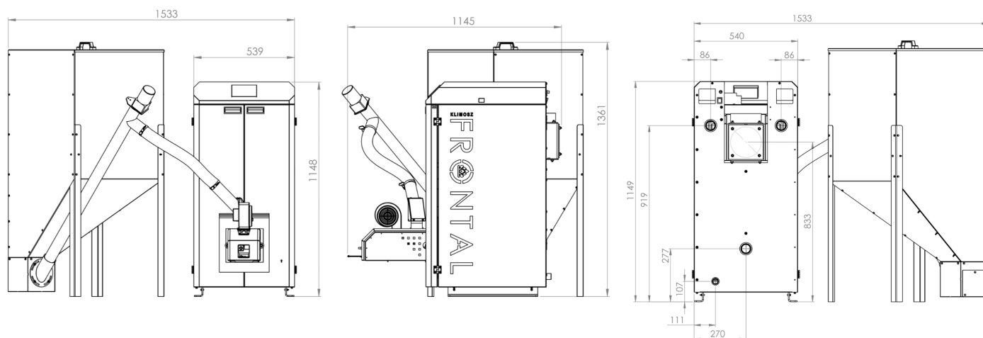
Frttonal 10-18 kW, w wersji z zewnętrznym zasobnikiem
