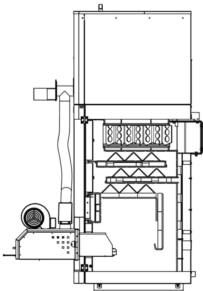
Rys. Przekrój kotła Frontal 15, w wersji z nadstawką
