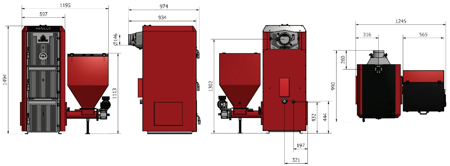
Rysunek poglądowy - COMBI S5 w wersji EKO z zasobnikiem 190L
