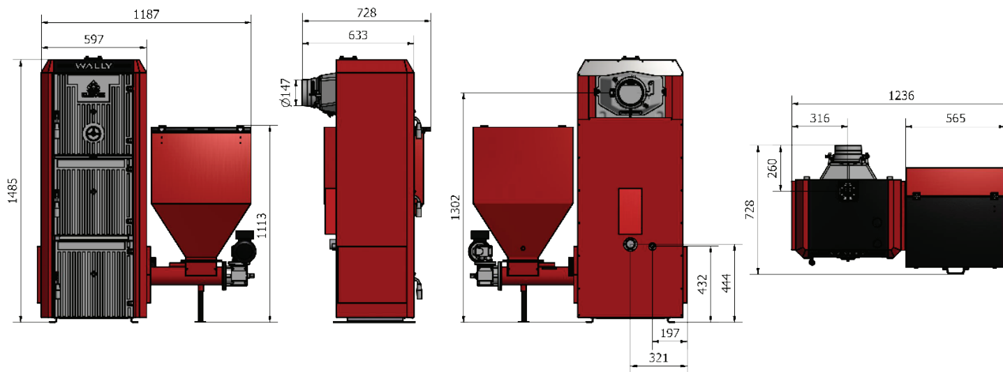
Rysunek poglądowy - COMBI S4 w wersji EKO z zasobnikiem 190L
