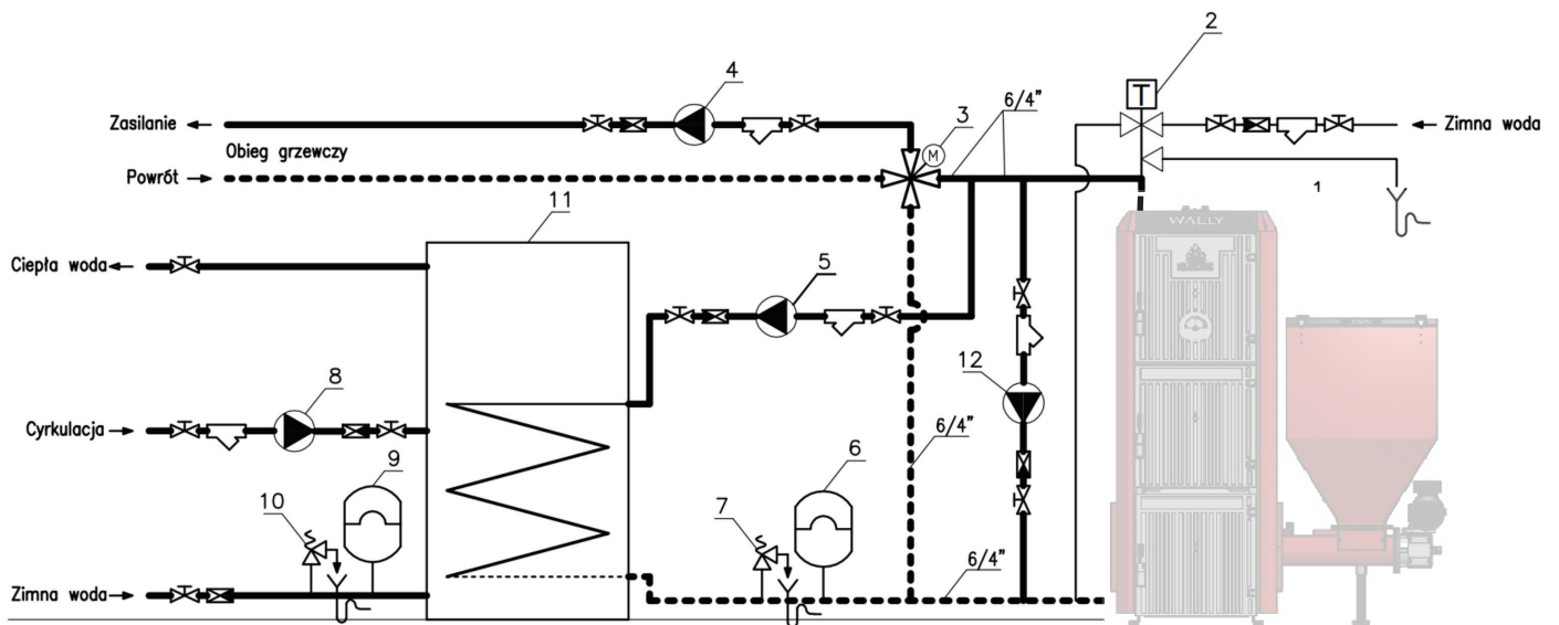
Rys. Schemat poglądowy montażu kotła COMBI S w układzie zamkniętym z zaworem DBV, zaworem czterodrogowym, pompą kotłową oraz bojlerem CWU
