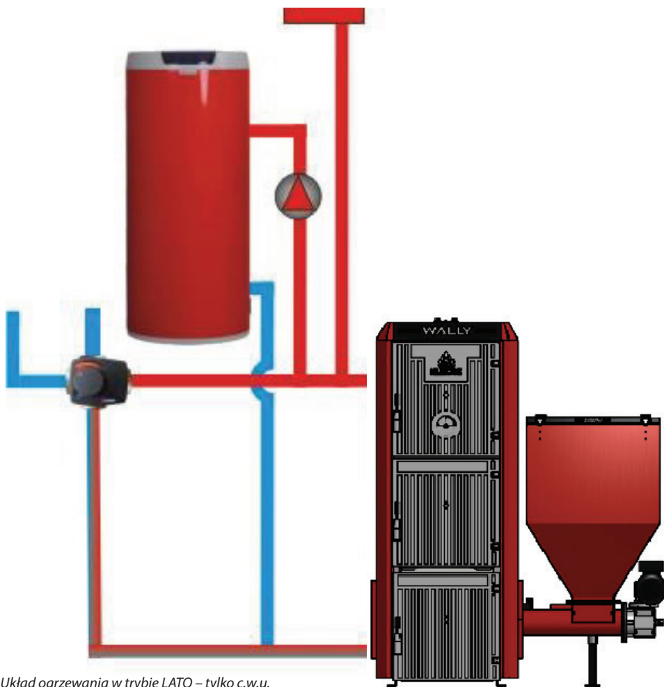
Układ ogrzewania w trybie LATO – tylko c.w.u.
