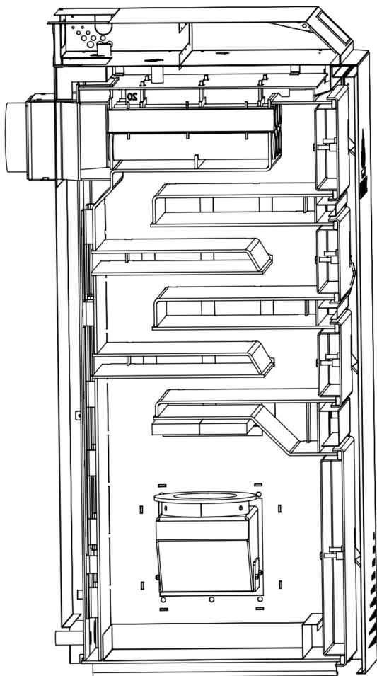
Rys. Poglądowy przekrój kotła (na przykładzie kotła LE25 w wersji NG)
