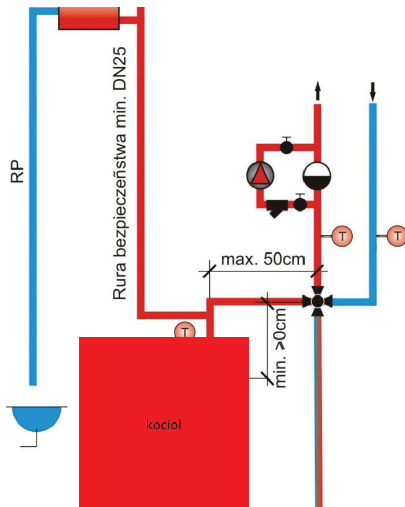
Rys. Schemat poglądowy umiejscowienia zaworu czterodrogowego oraz jego odległości maksymalnych od kotła
