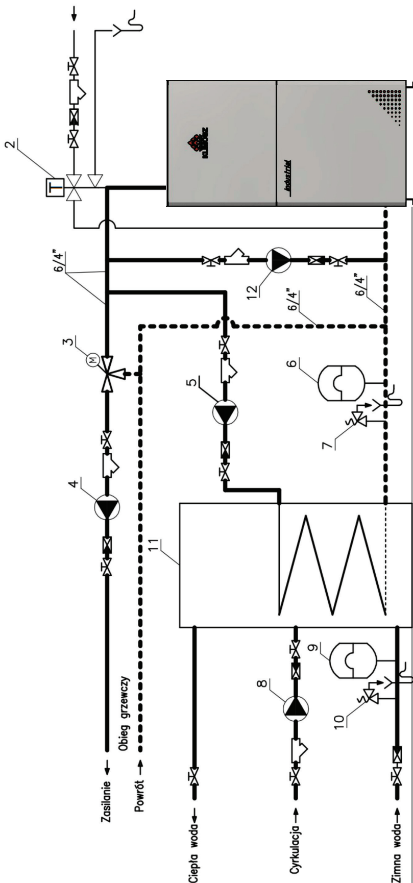
Rys. Schemat poglądowy montażu kotła LE PELET w układzie zamkniętym z zaworem DBV, zaworem trójdrogowym, pompą kotłową oraz boilerem CWU.
