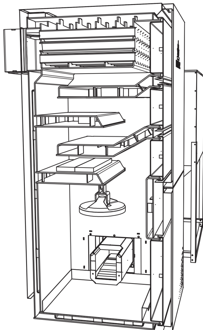
Rys. Przekrój kotła (na przykładzie modelu 75)
