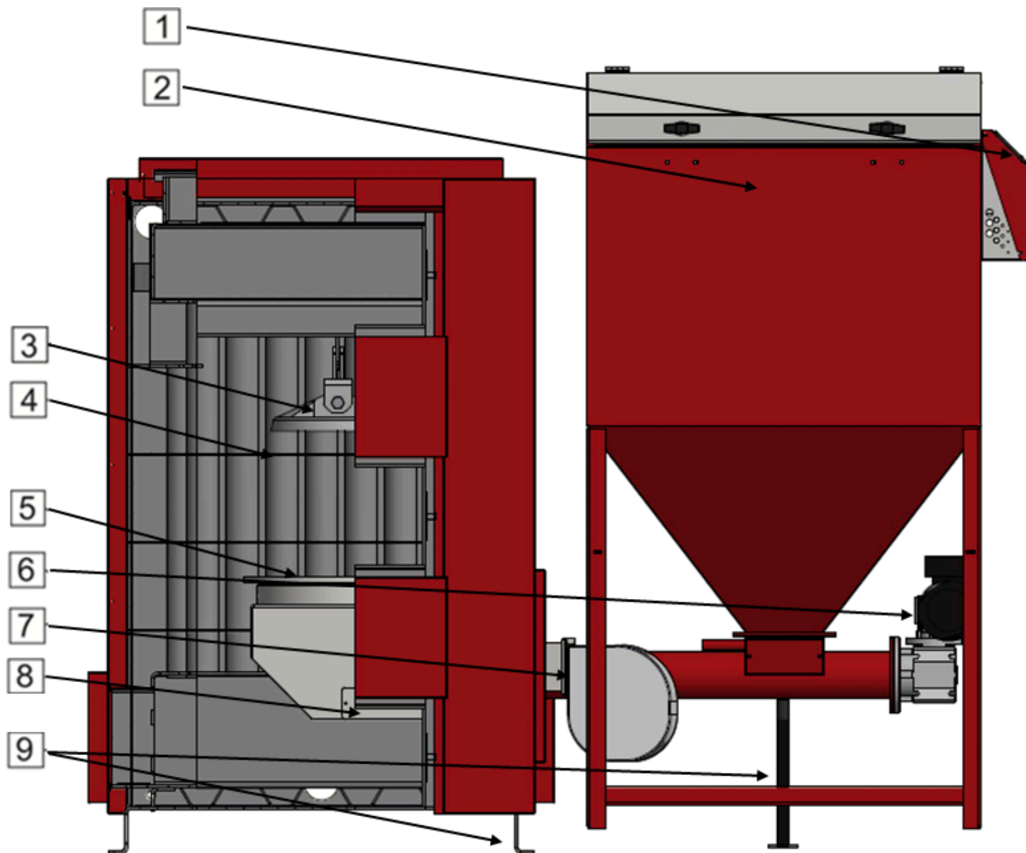
RYSUNEK POGLĄDOWY KONSTRUKCJI KOTŁA KLIMOSZ MAXI:
