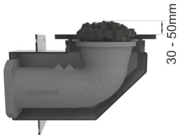
Poglądowe uytuowanie paliwa względem palnika retortowego podczas pracy kotła
