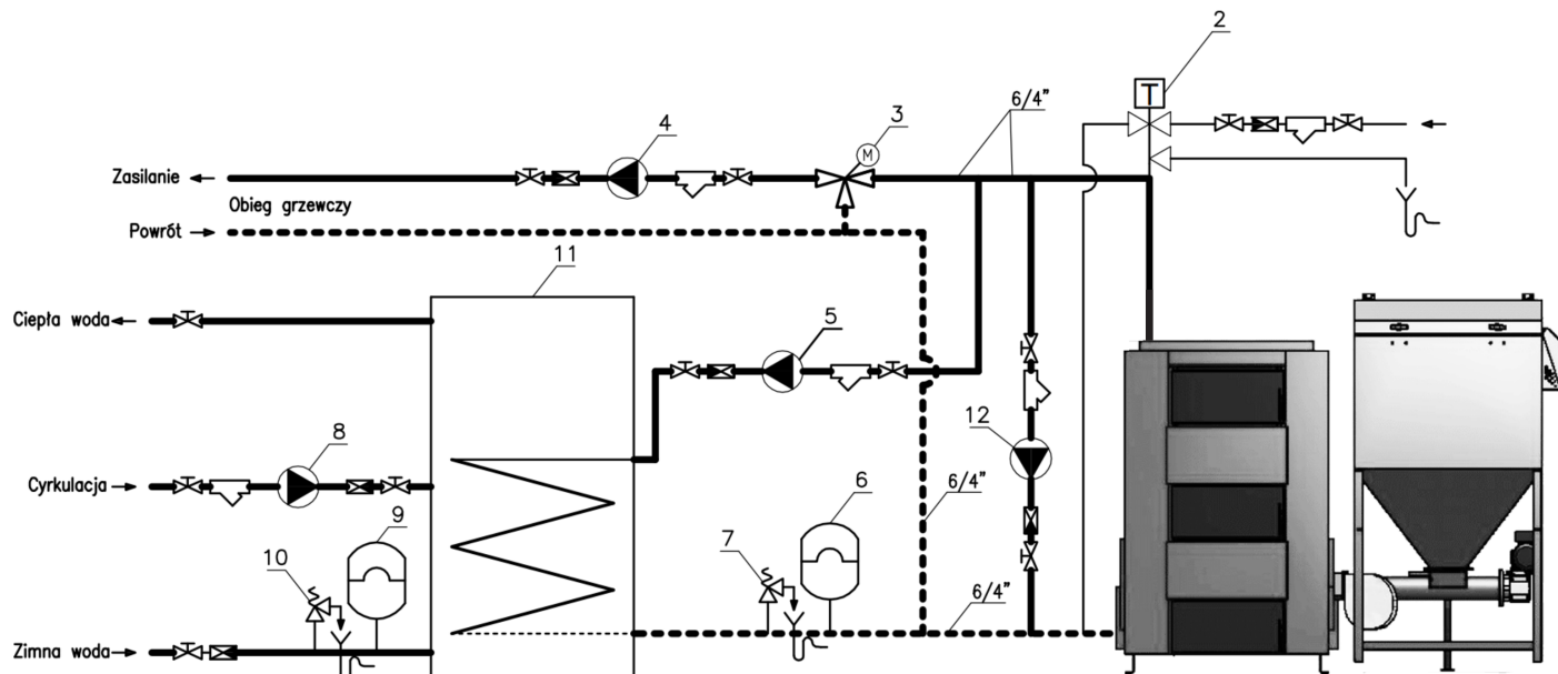
Rys. Schemat poglądowy montażu kotła MAXI w układzie zamkniętym z zaworem DBV, zaworem trójdrogowym, pompą kotłową oraz bojlerem CWU.
