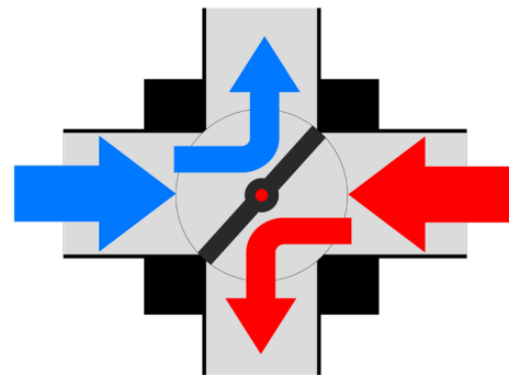
Rys. Pełne zamknięcie siłownika zaworu czterodrogowego
