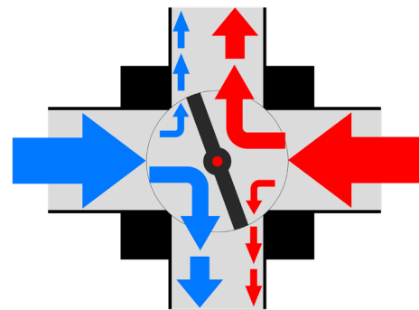
Rys. Siłownik zaworu czterodrogowego podczas normalnej pracy
