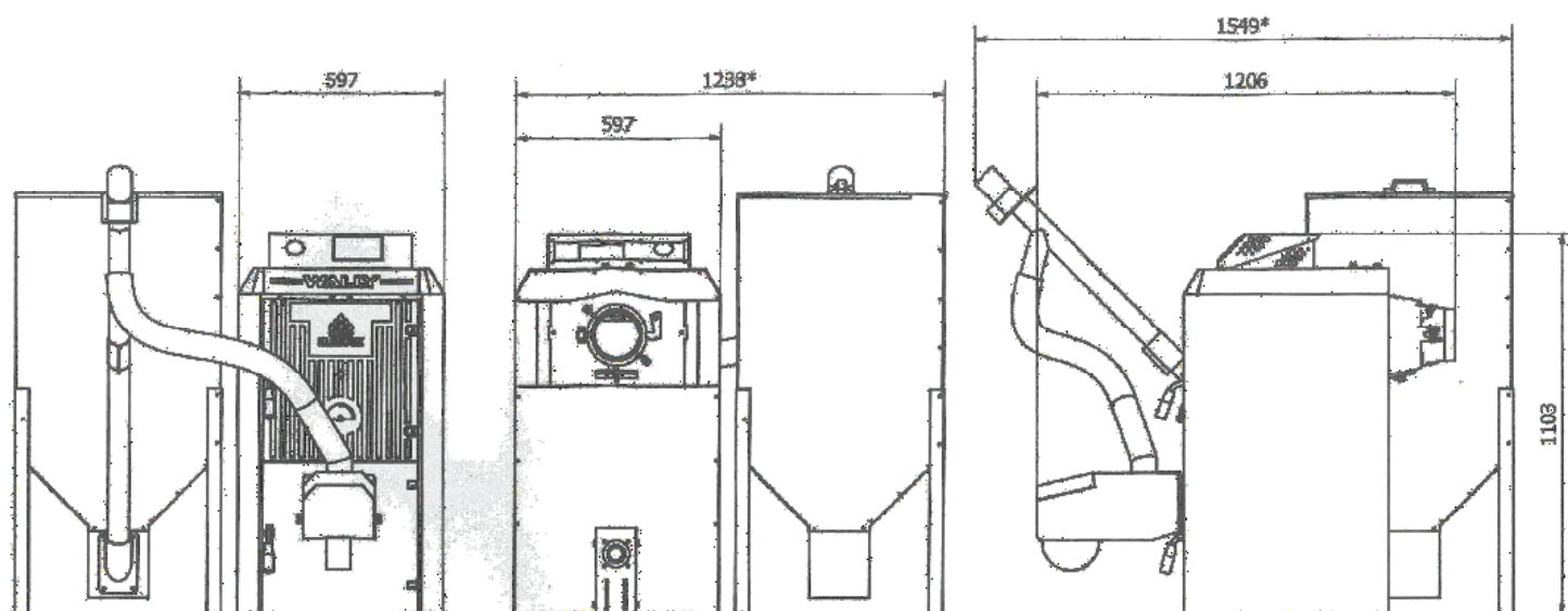
Rys. Wymiary kotła UNIPELET 45
