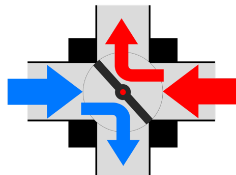
Rys. Pełne otwarcie siłownika zaworu czterodrogowego
