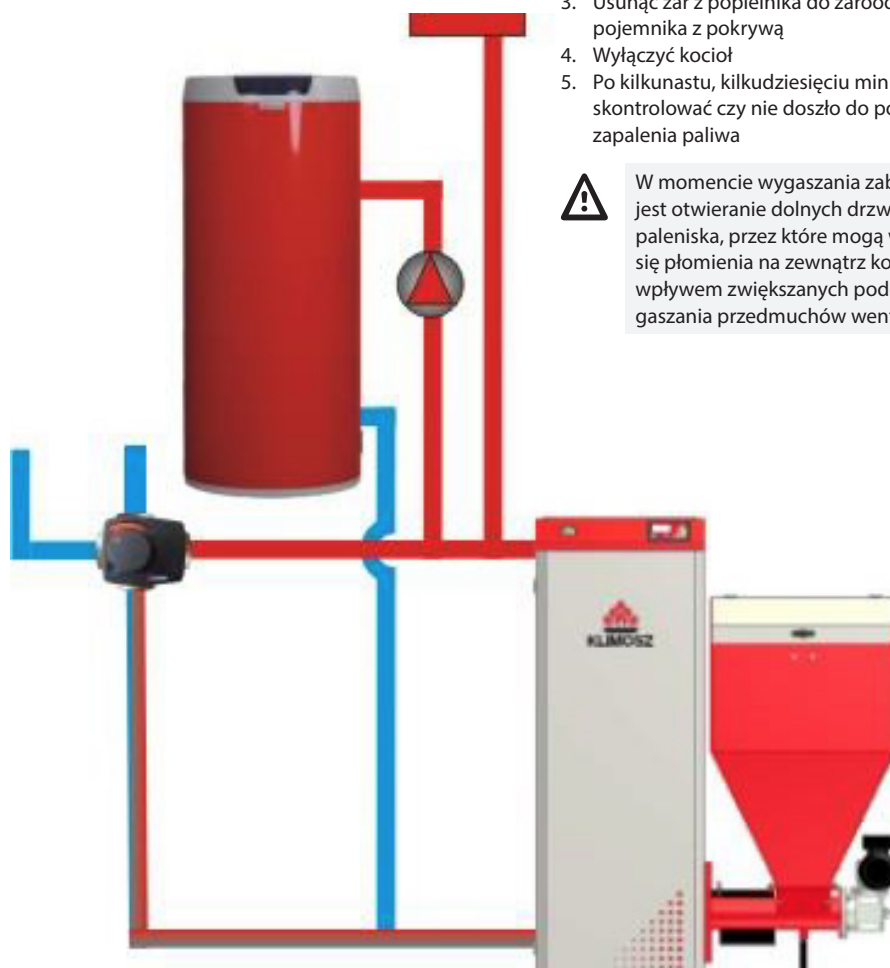
Układ ogrzewania w trybie LATO – tylko c.w.u.
