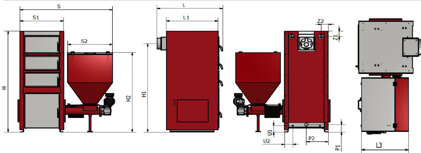
seria LE z palnikiem retortowym - wersja NG
